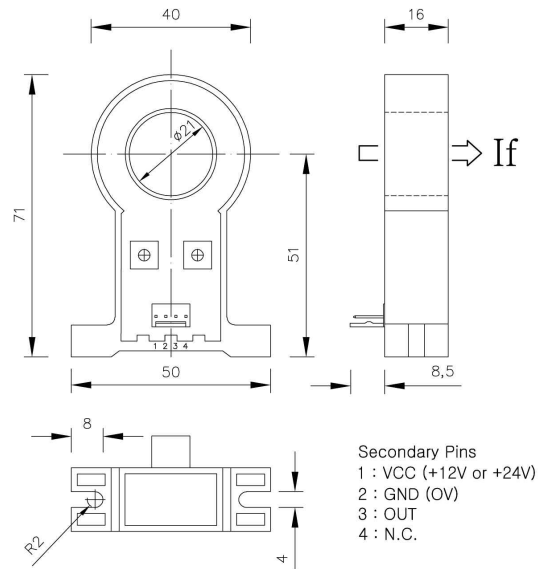
TS-타입 전류스위치 DIMENSIONS(mm)
